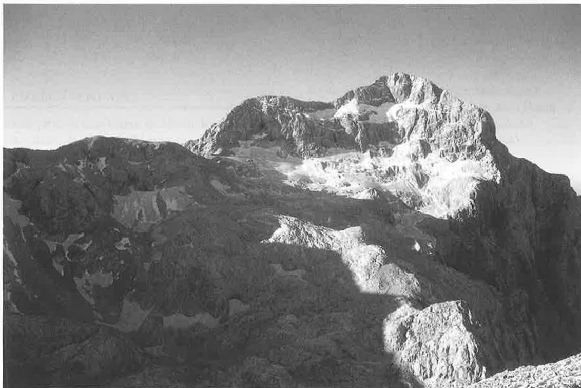
Preučevanje Triglavskega ledenika, ki se je začelo že leta 1946, je verjetno najstarejši stalni slovenski znanstveni projekt. Leta 2001 se Triglavski ledenik po dolгих letih, predvsem zaradi debele snežne odeje, ni zmanjšal (fotografija: Matija Zorn, 16. 10.).
